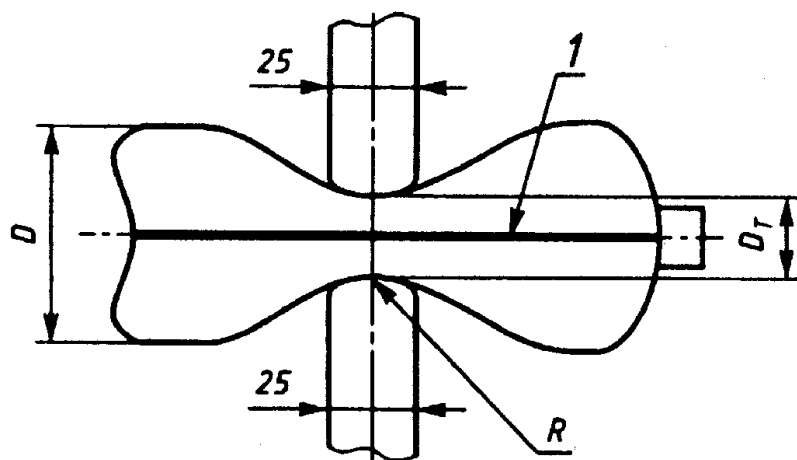
1 — сварной шов; R=12,5 ; D_t = D/3 ; D_t — расстояние после испытаний; D — наружный диаметр цилиндра
