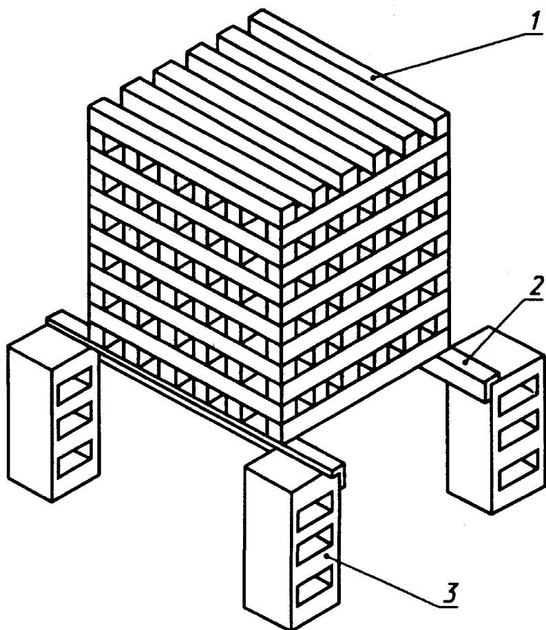
1 — деревянный брусок; 2 — стальной уголок; 3 — бетонный (металлический) блок
